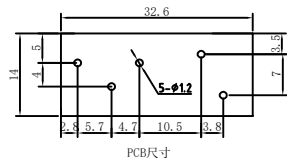
PCB尺寸
